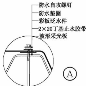
压型钢板复合保温卷材防水屋面(机械固定1)玻璃钢采光带
