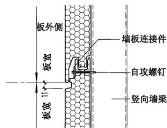
③ 竖向连接
