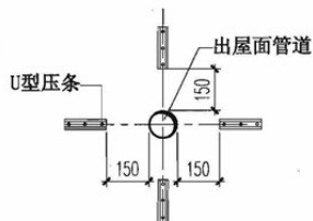
U型压条平面布置示意(二)
