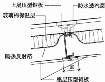
屋面底层板纵向搭接
