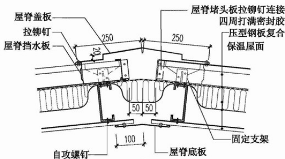
⑬ 屋脊
