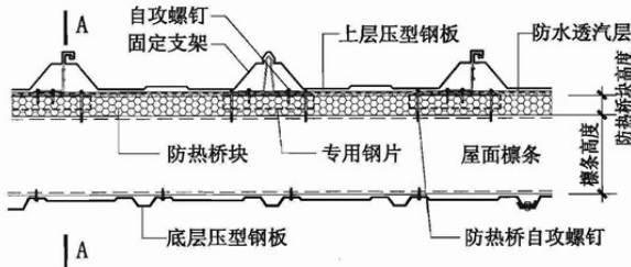
屋面横向连接
