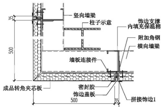
⑤ 阳角
