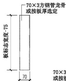
墙板竖向龙骨
