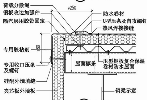
⑦ 山墙封口
