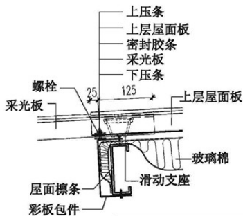
15 采光板纵向搭接
