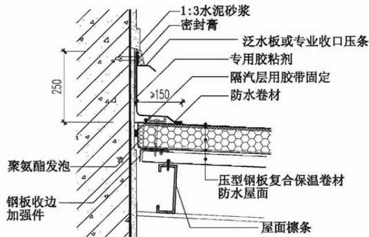
⑩ 高低跨
