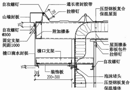
③ 山墙挑檐
