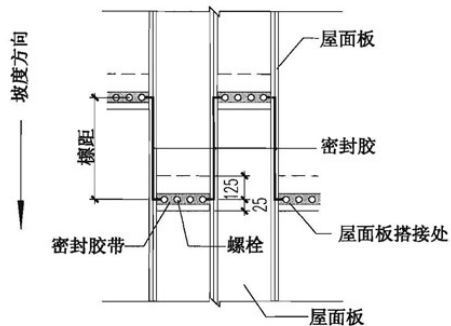
屋面板搭接及打胶示意平面图
