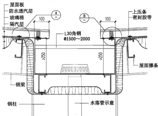
⑧ 内天沟
