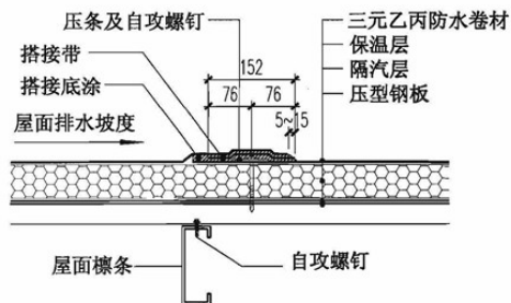
三元乙丙防水卷材屋接缝固定做法
