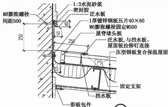
20 高低跨
