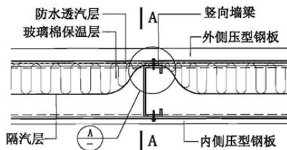
墙体横向连接
