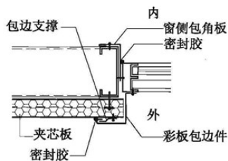
⑪ 窗侧
