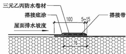
三元乙丙防水卷材标准搭接做法
