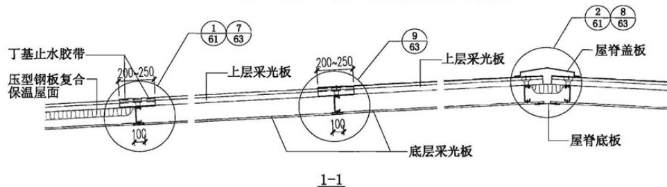
屋10、屋11、屋12-采光板复合屋面构造
