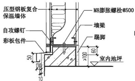
⑧ 墙脚
