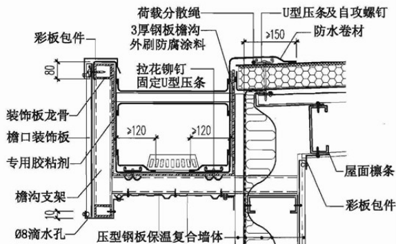
②0 外檐沟
