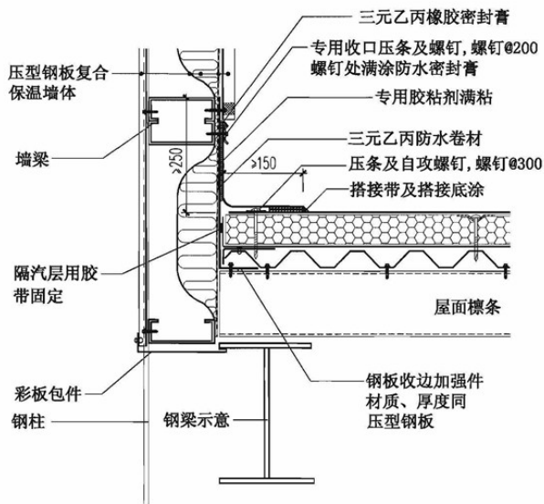
高低跨
