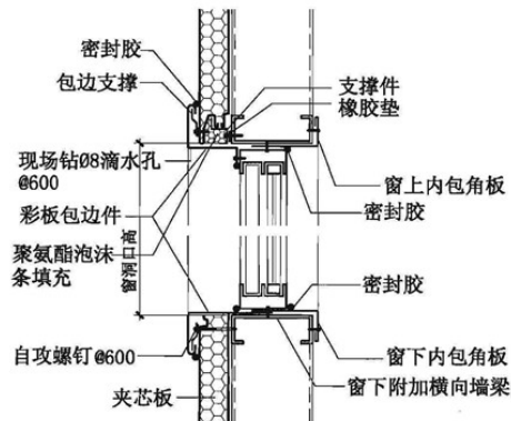
⑩ 窗顶、窗底
