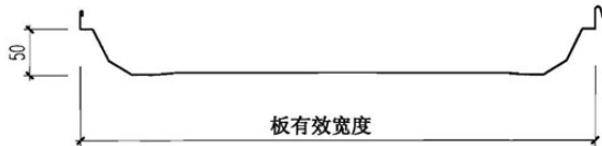
直立缝锁边连接屋面板
