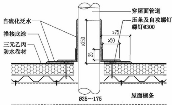
③ 穿屋面管道
