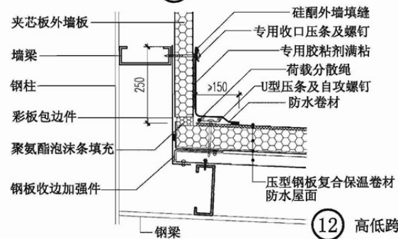
压型钢板复合保温卷材防水屋面(机械固定1)高低跨
