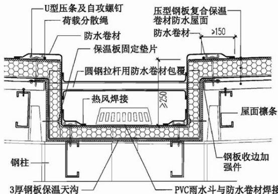
①9 外檐沟
