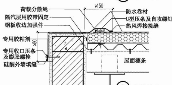
⑧ 山墙封口
