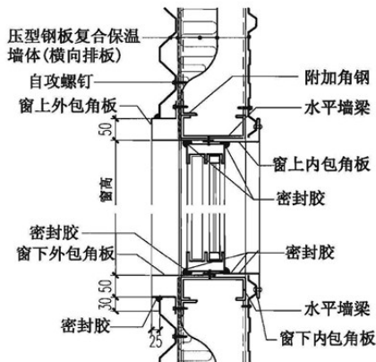
⑦ 窗顶、窗底
