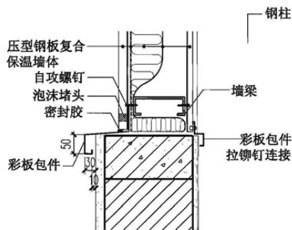
⑥ 墙脚
