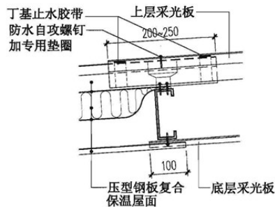
⑦ 纵向搭接
