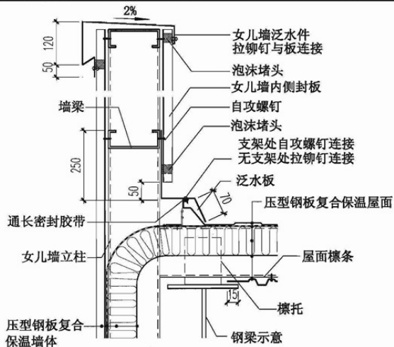
⑫ 山墙女儿墙
