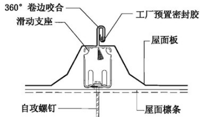
锁边示意
