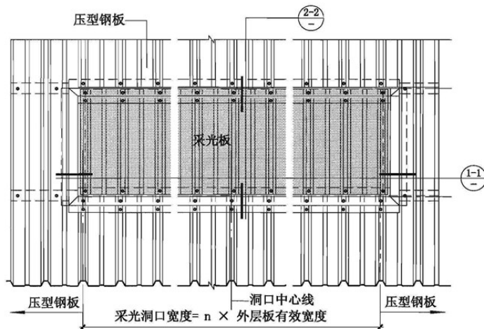
图6、7-波形树脂采光板墙体(镶嵌式)立面示意
