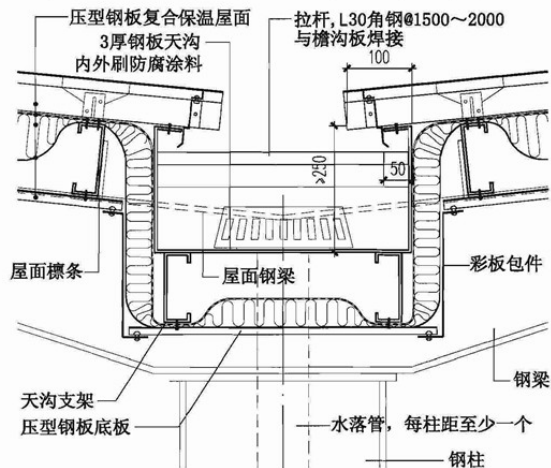
⑧ 柱间内天沟
