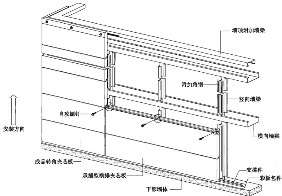
图4A-夹芯板承插型墙体(横向排板)构造
