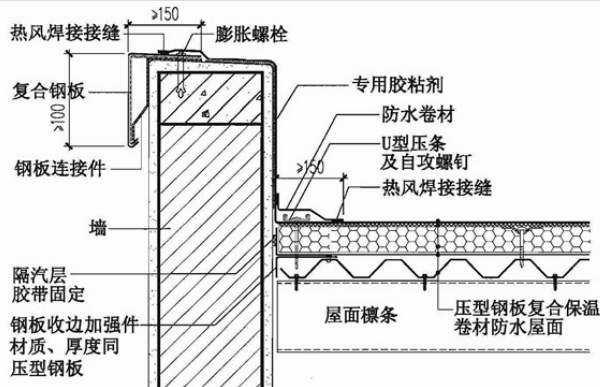
⑤ 山墙封口
