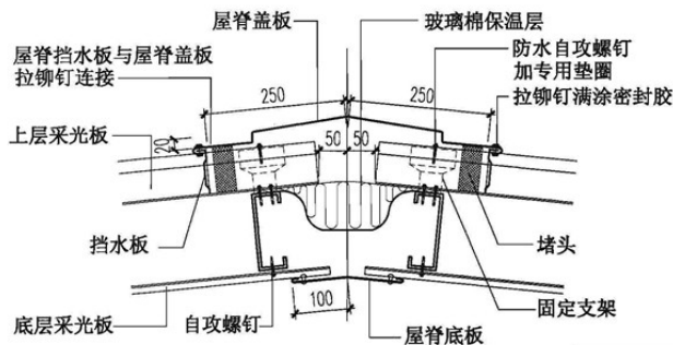
⑧ 屋脊
