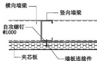
① 墙板与墙梁连接
