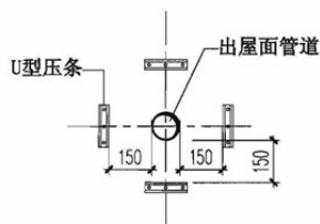
U型压条平面布置示意(一)
