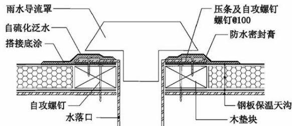
④ 水落口做法
