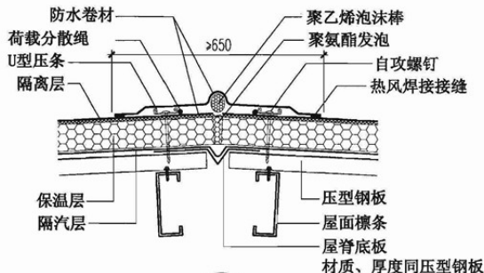
③ 屋脊
