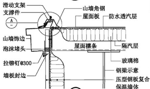
④ 山墙
