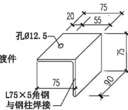
角钢连接件大样图
