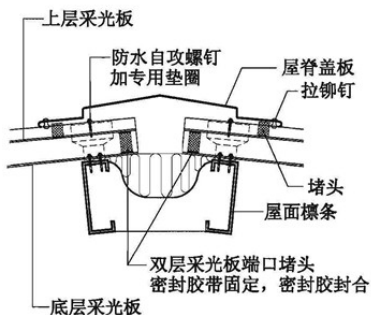
② 屋脊
