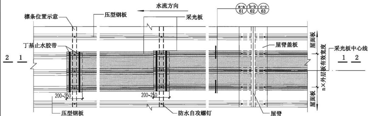
屋10、屋11、屋12-采光板复合屋面构造
