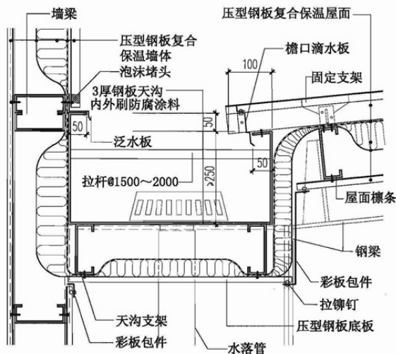
10 高低跨内天沟
