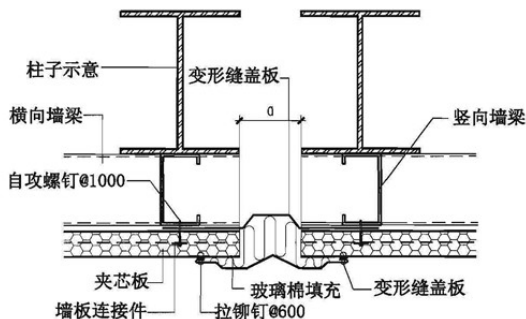
④ 变形缝
