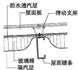
屋面板纵向连接
