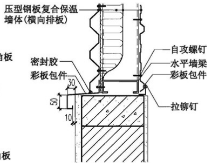
⑨ 外墙脚
