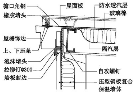
③ 单坡屋脊
