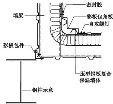
③ 阴角
