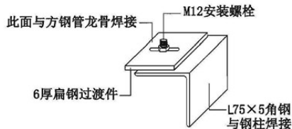
方钢管龙骨端部连接大样图
