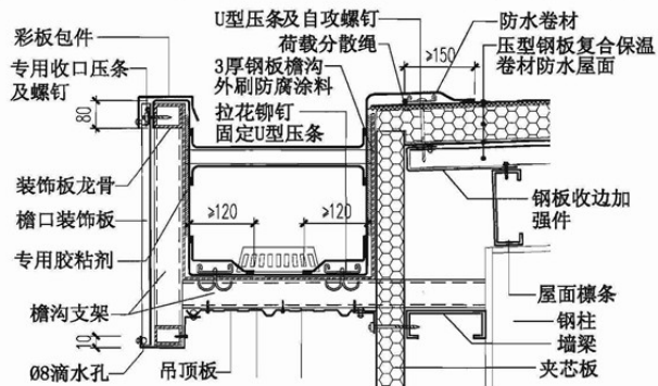
①9 外檐沟
