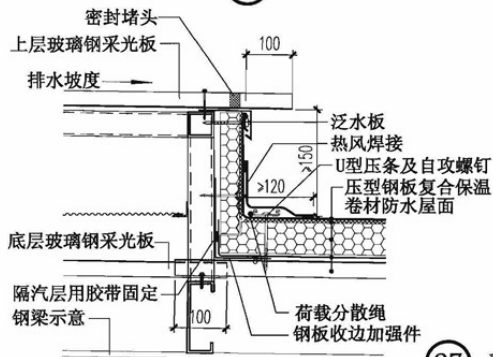
27 采光带
