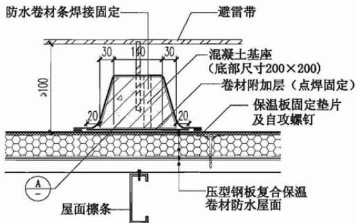
④ 屋面避雷带
