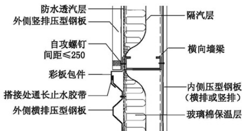
C 横排墙板与竖排墙板纵向连接(二)
