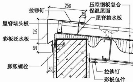
16 单坡屋脊
