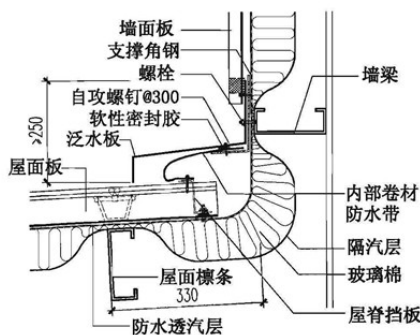
12 高低跨
