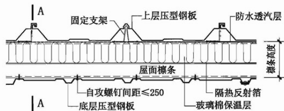
屋面横向连接
