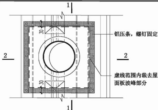
出屋面管道平面图
