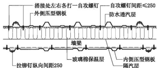
墙体横向连接
