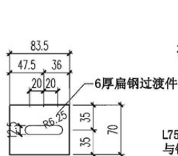
扁钢过渡件大样图
