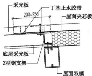
⑥ 纵向搭接
