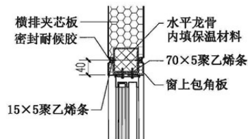
① 窗顶
