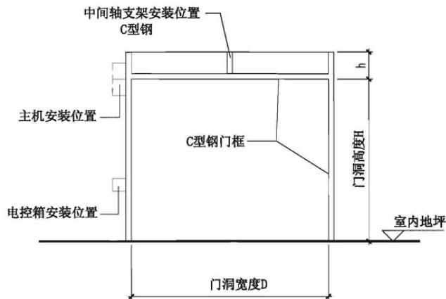
钢门框立面示意图
