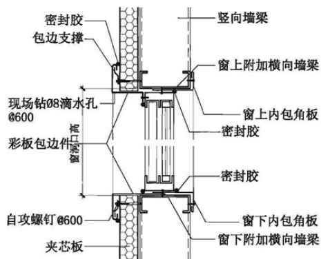
⑨ 窗顶、窗底
