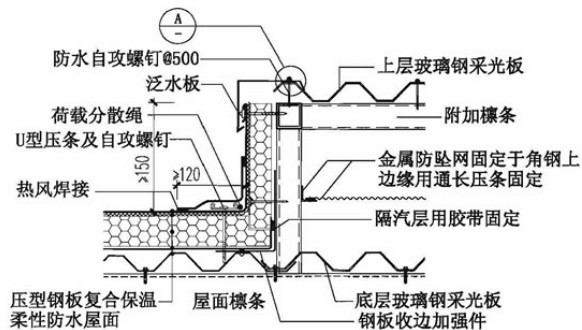
25 采光带
