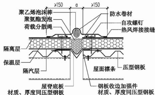
① 水平变形缝
