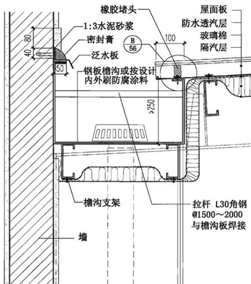
⑦ 女儿墙内檐沟
