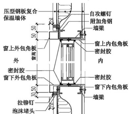
⑤ 窗顶、窗底
