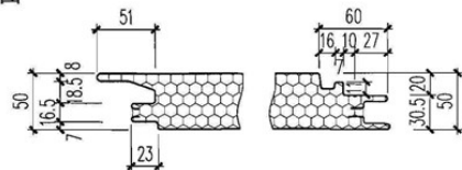
夹芯板端部详图 (以50板厚为例)
