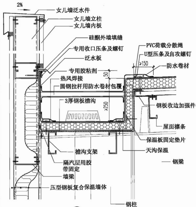
⑰ 女儿墙内檐沟
