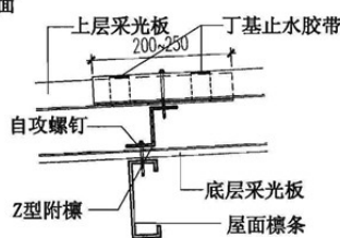
⑤ 纵向搭接
