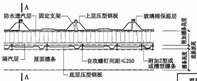
屋面横向连接
