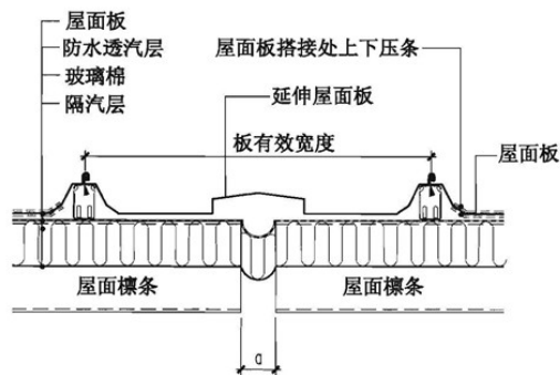
⑨ 变形缝
