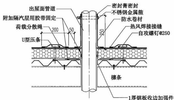
30 出屋面管道
