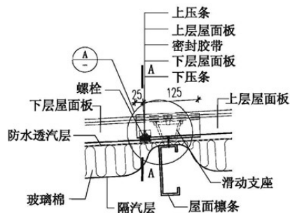
屋面板纵向搭接
