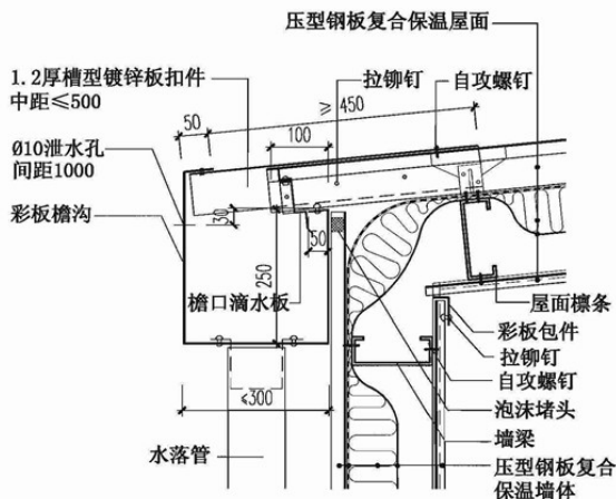
④ 外檐沟
