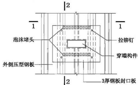
构件穿墙做法(一)
