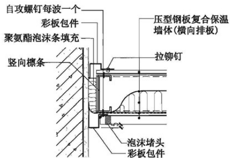
⑤ 与混凝土墙连接
