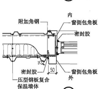
⑦ 窗侧
