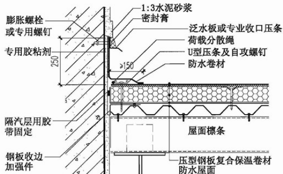
⑨ 高低跨
