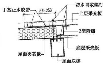
③ 纵向搭接
