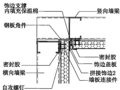
⑥ 阴角
