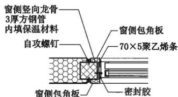
③ 窗側
