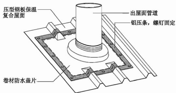
卷材防水盖片示意图
