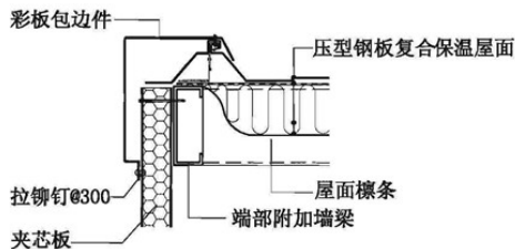
⑧ 山墙
