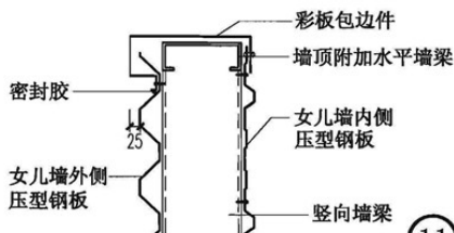
⑪ 女儿墙顶
