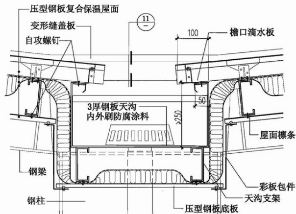
9 内天沟
