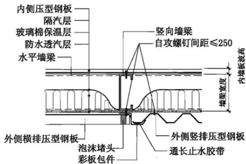
A 横排墙板与竖排墙板水平连接
