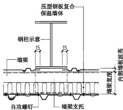
② 遇柱处
