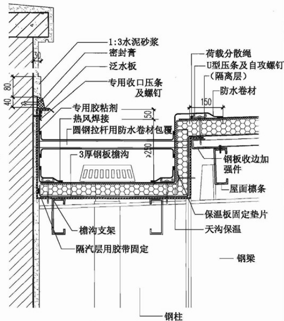
⑱ 女儿墙内檐沟
