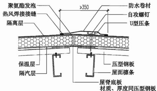
② 屋脊
