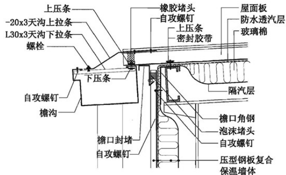
① 外檐沟
