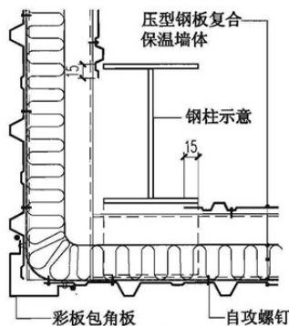
① 阳角
