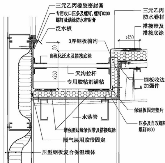
⑤ 女儿墙内檐沟
