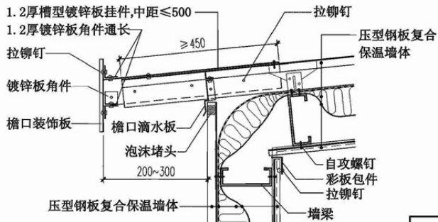
② 檐口
