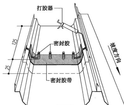
屋面板搭接处打胶方式
