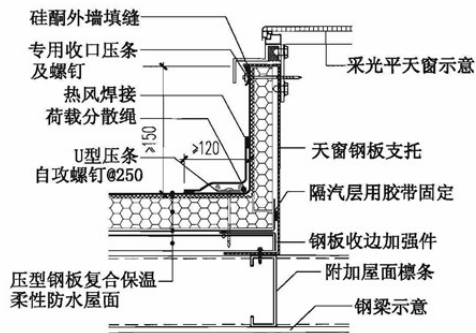
28 天窗
