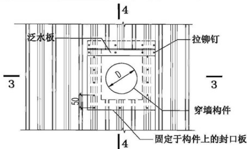
构件穿墙做法(二) (用于 D \geq 1000 )
