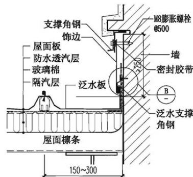
11 高低跨
