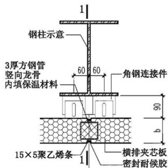
竖向龙骨与板拼接
