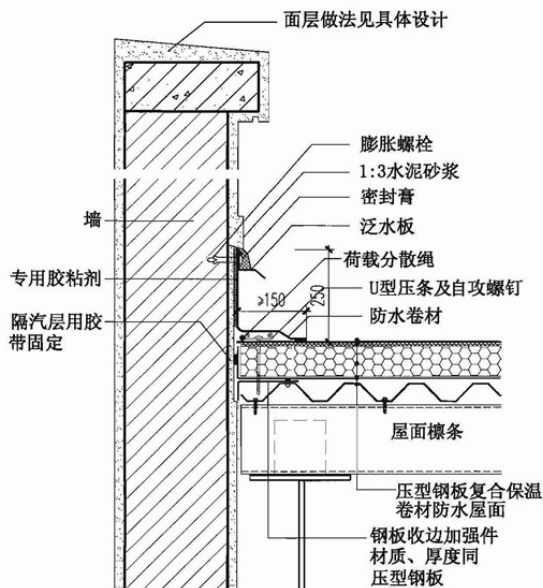
⑯ 女儿墙
