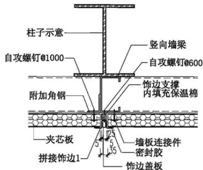
② 横向连接
