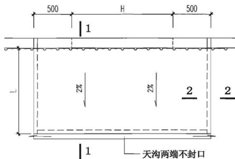
雨棚平面图
