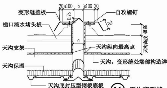
11 天沟变形缝
