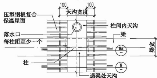
内天沟平面图
