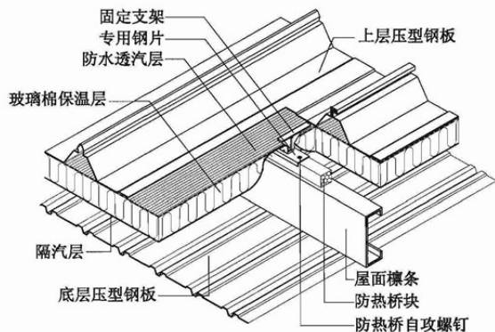
压型钢板复合保温屋面隔热桥构造
