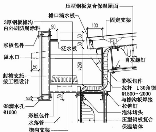
⑤ 外檐沟
