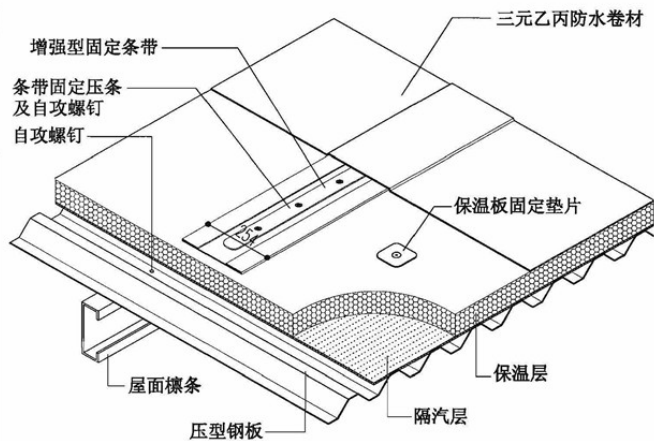
三元乙丙防水卷材屋面(机械固定)做法
