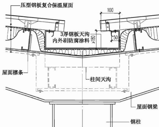
⑧a 遇梁处内天沟
