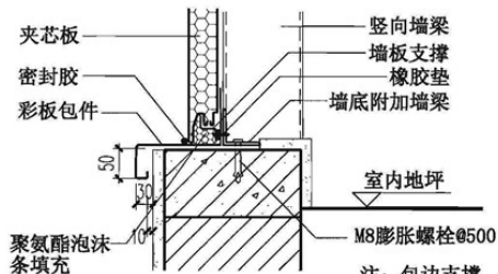
⑫ 地脚
