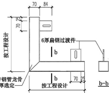
墙板转角水平龙骨
