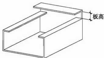
① A 天沟变形缝处端部构造
