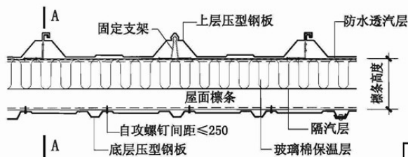
屋面横向连接
