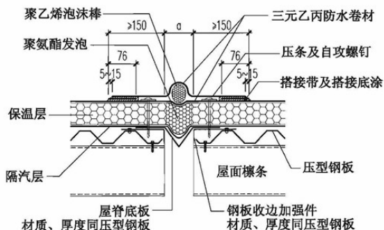
屋面变形缝
