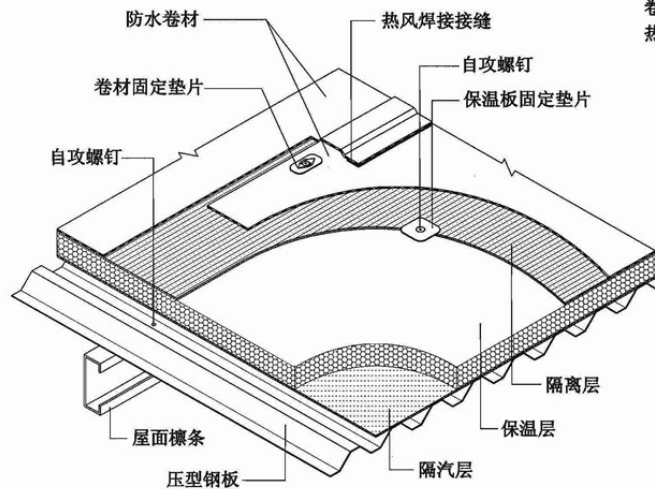
屋6-压型钢板复合保温卷材防水屋面(机械固定1)构造
