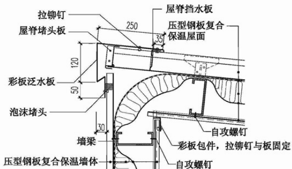
15 单坡屋脊
