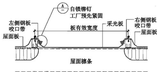
14 采光板横向搭接
