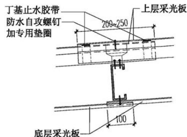
⑨ 纵向搭接
