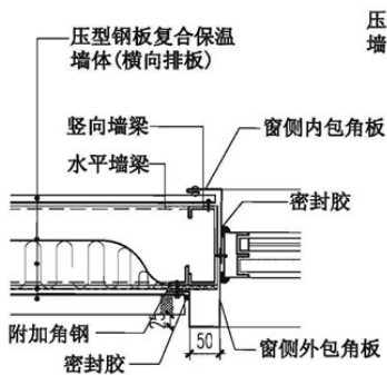
⑧ 窗侧
