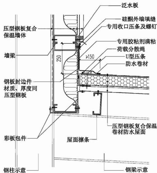
14 高低跨
