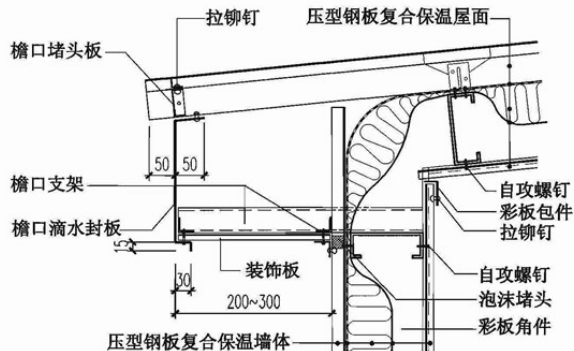
① 檐口
