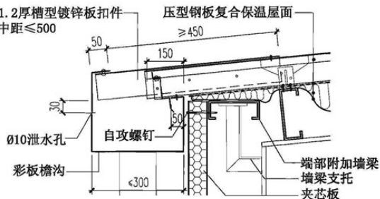
⑦ 檐口
