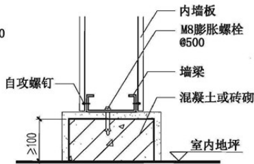
⑨ 内墙墙脚
