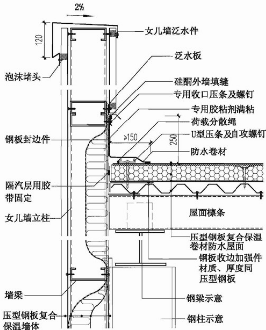
⑮ 女儿墙
