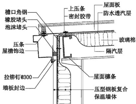
② 檐口
