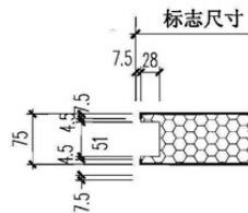
Ⓑ 75厚墙板端部详图
