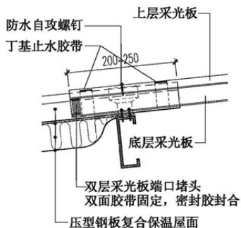
① 纵向搭接
