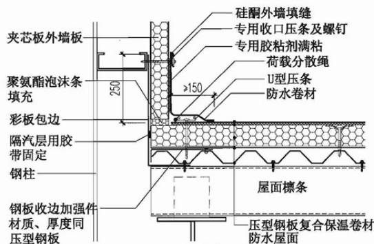
⑪ 高低跨
