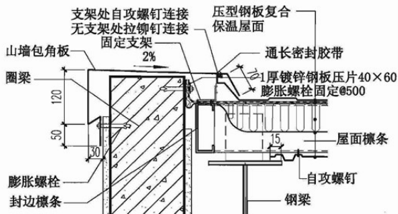
18 山墙
