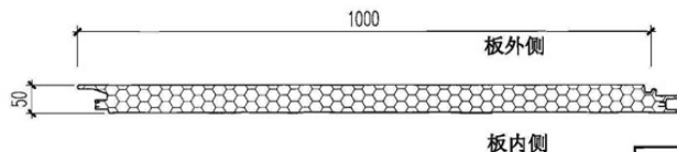
承插型夹芯板(横向排板)板型
