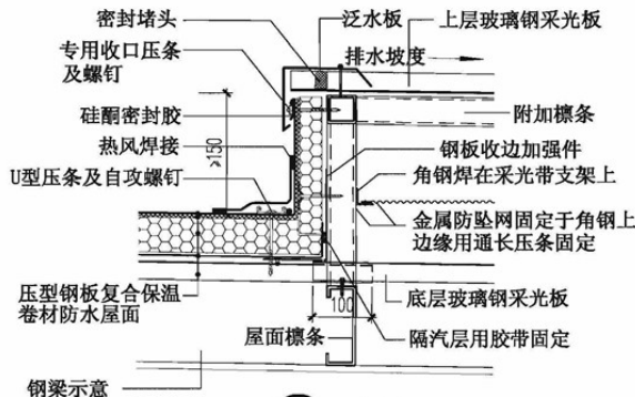
26 采光带
