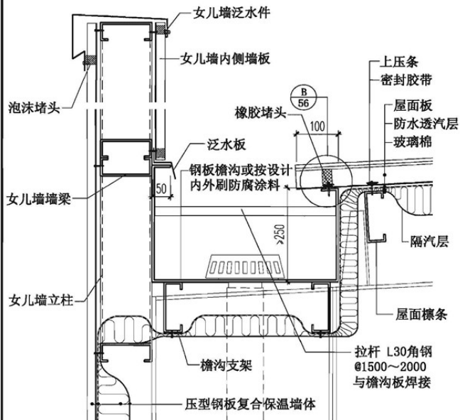
⑥ 女儿墙内檐沟
