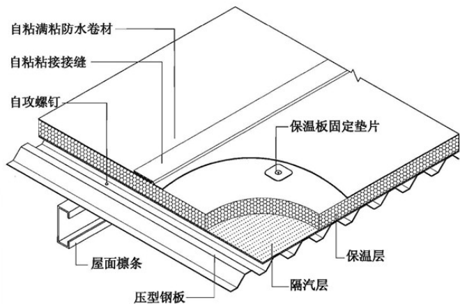
屋7-压型钢板复合保温卷材防水屋面(满粘固定)构造
