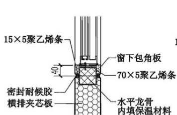
② 窗底
