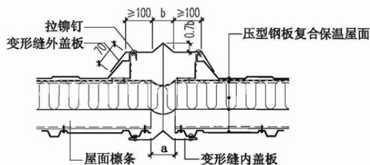
⑭ 屋面变形缝
