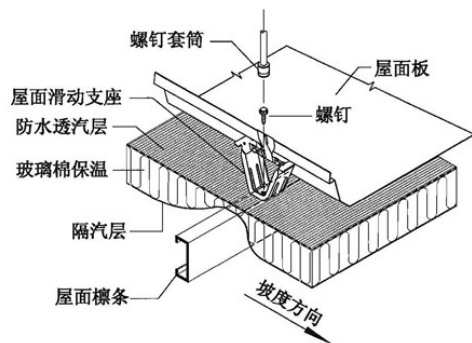
压型钢板复合保温直立缝滑动屋面构造
