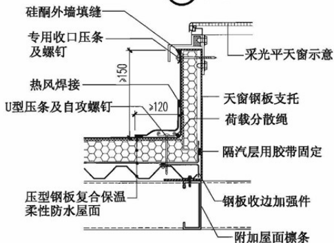
29 天窗
