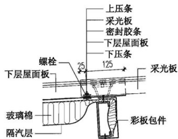
15 采光板纵向搭接
