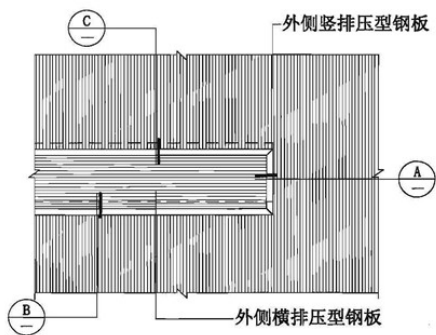
立面示意
