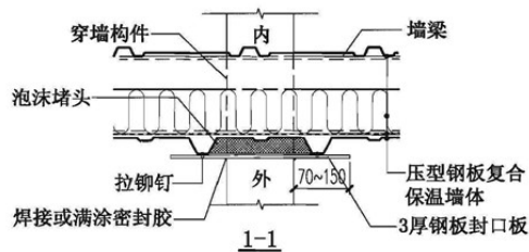
构件穿墙做法(一)
