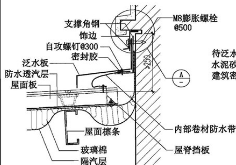
10 高低跨
