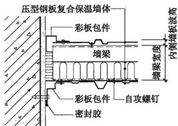
④ 与混凝土墙连接
