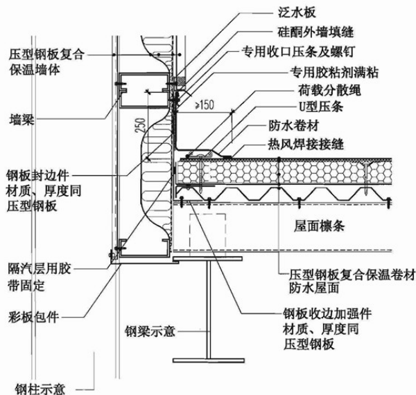
13 高低跨
