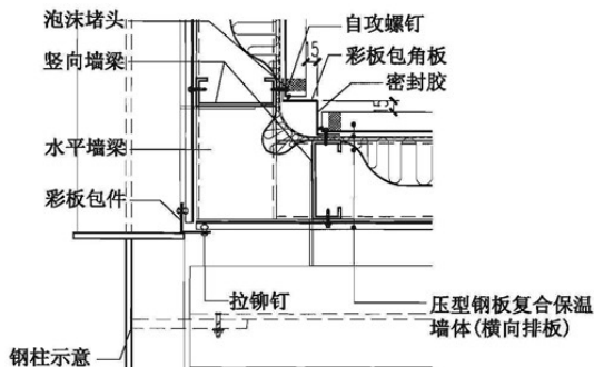
④ 阴角
