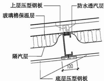
屋面底层板纵向搭接
